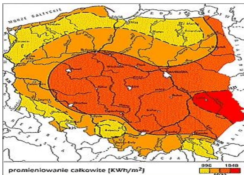
Rys. 2.3. Promieniowanie całkowite w Polsce
