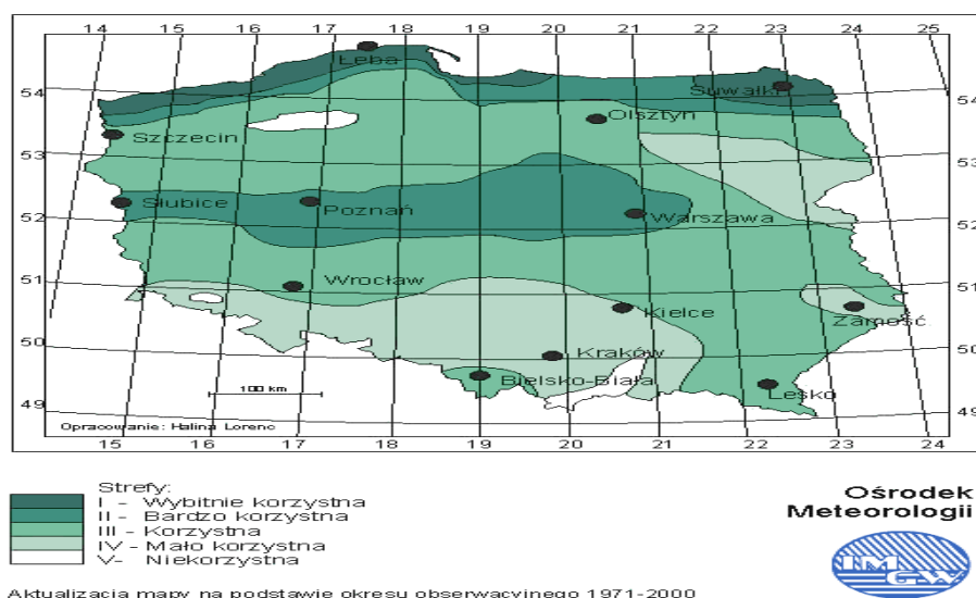
Rys. 2.4. Strefy energetyczne wiatru w Polsce
