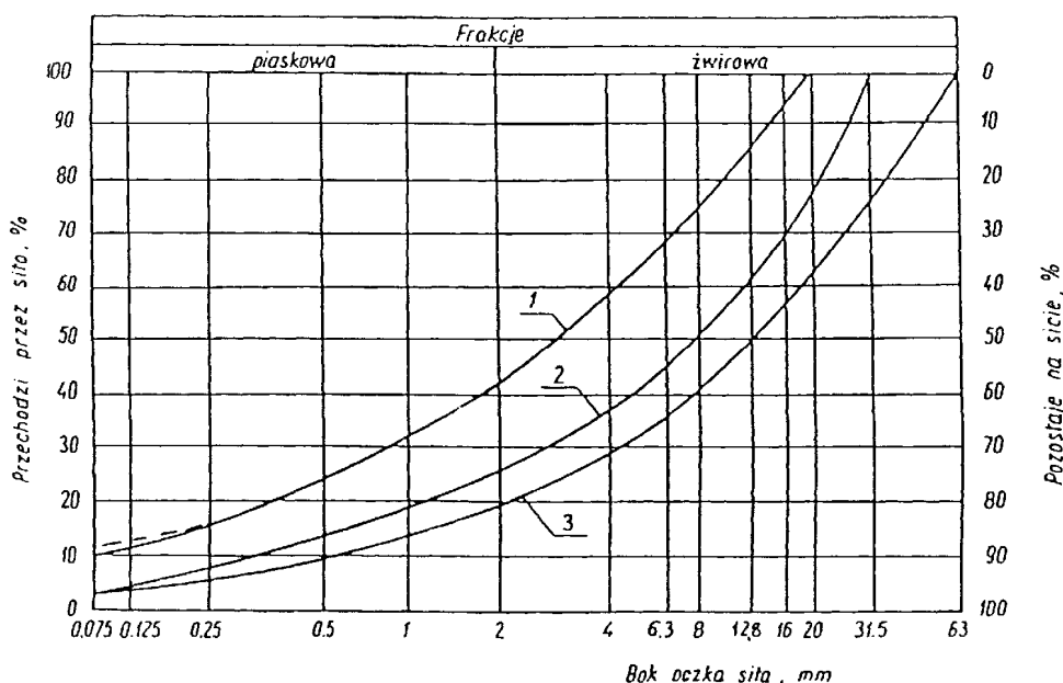
Rysunek 1. Pole dobrego uziarnienia kruszyw przeznaczonych na podbudowę wykonywane metodą stabilizacji mechanicznej 1-2 kruszywo na podbudowę zasadniczą (górną warstwę) lub podbudowę jednowarstwową kruszywo na podbudowę pomocniczą (dolną warstwę)
